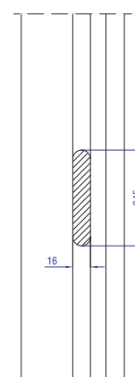
Sectiune Montaj Canat
