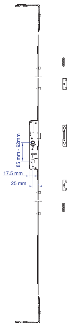
Sectiune Montaj Canat
